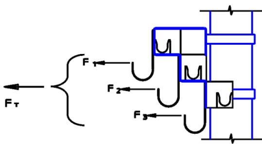
Figura 1 - Detalhe para execução do ensaio
